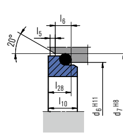
G6 EN 12756
