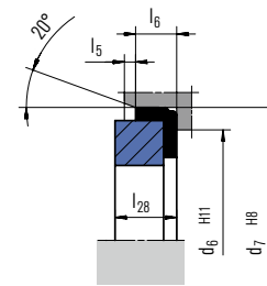
G60 EN 12756
