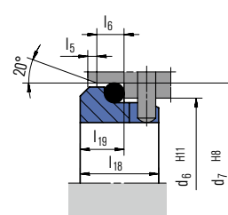
G16 (EN 12756)
