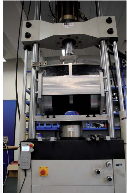
Sideværts stress test af SES 6000 chok ophæng
