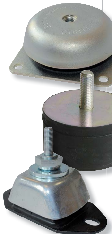
SCHWINGMETALL® og WILLBRANDT elBe ophæng med spindel
