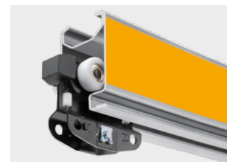
Löpvagnen löper inne i profilen
