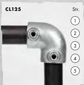
Bøjning (90°)
