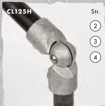
Justerbar bøjning (202°)
