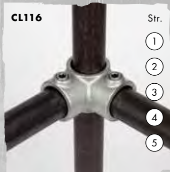
3-vejs hjørne (90°)
