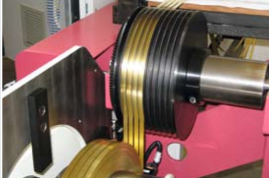
Dünmbandwickelsystem: Wickeln mit konstantem Aufwickelwinkel Thin gauge recoiling system: Rewinding with constant recoiling angle
