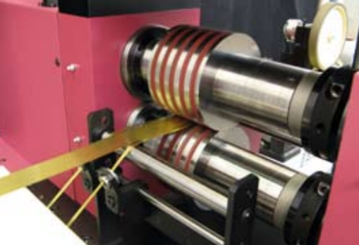
Schneiden mit Gummiauswerferringen Cutting by using rubber stripper rings
