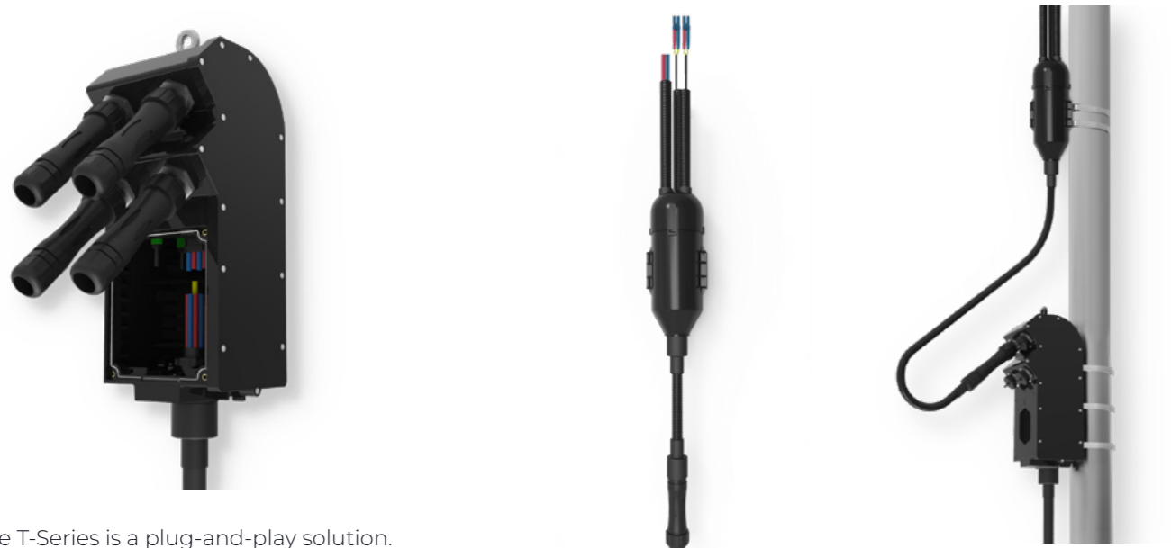
Conduit pest-proof hybrid drop
