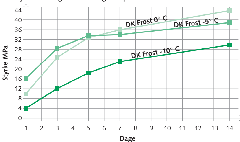
Styrkeudvikling ved forskellige temperaturer
