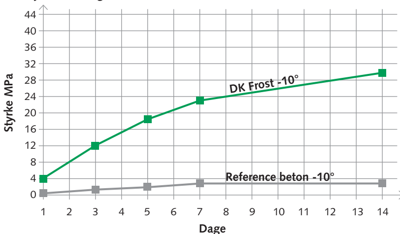
Styrkeudvikling ved -10° C
