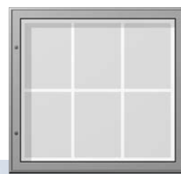
6 x A4 (Portrait) Udvendigt mål: 815 x 760 mm Lysmål: 704 x 651 mm
