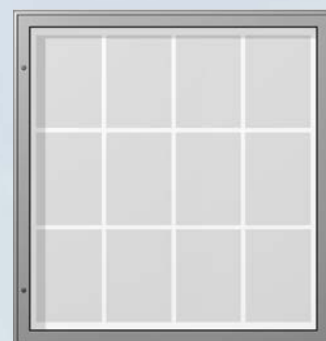
12 x A4 (Portrait) Udvendigt mål: 1000 x 1085 mm Lysmål: 889 x 976 mm
