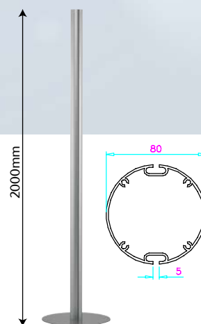
ODS 2000mm - ingen top Ø450mm fodplade
