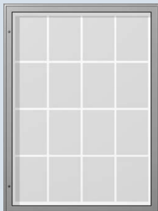
16 x A4 (Portrait) or A0 Udvendigt mål: 1000 x 1405 mm Lysmål: 889 x 1296 mm
