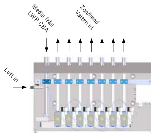
Lagafors® DSA II, automatisk distributionssatellit.
