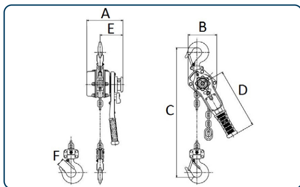
Måttskiss KITO Spaklyftblock LB OLL
