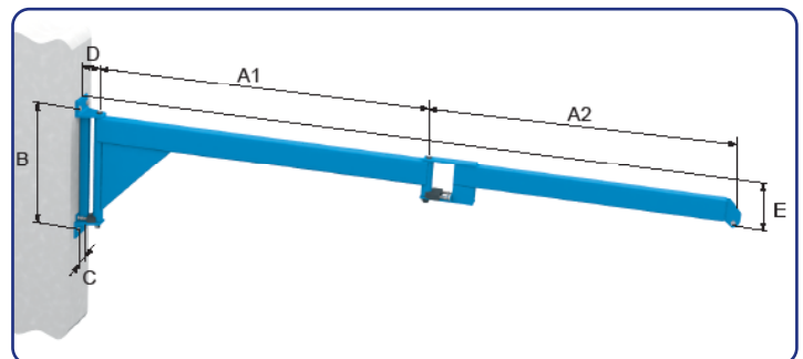
Måttskiss Väggknäckarm Hymer
