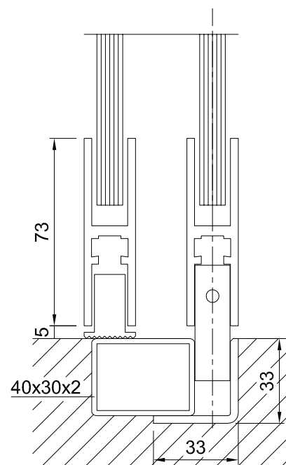
Gulvkonstruktion
