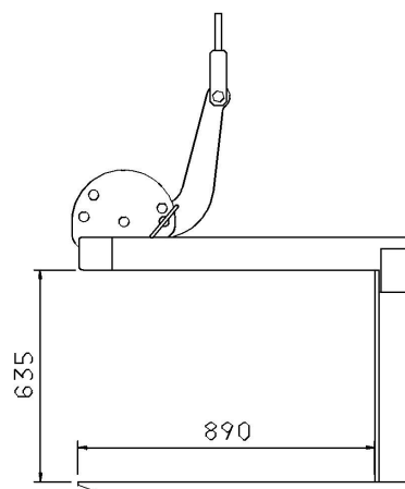
GPV2 lastet med 900 mm plader vandret
