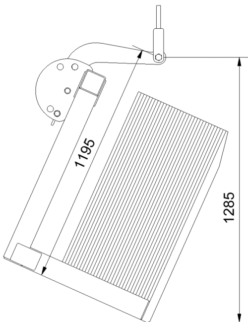
GPV2 lastet med 900 mm plader vandret
