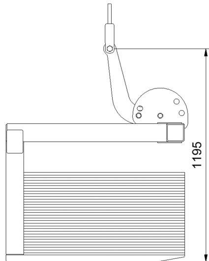
Gipspladevender GPV2 1500 1,5T
