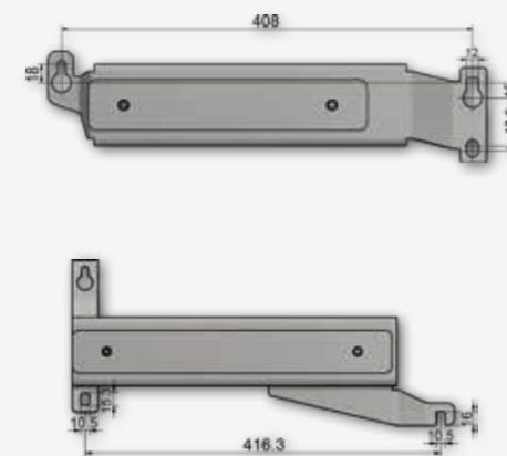
KONSOL Galvaniserad BevoBox™ höger Scania
