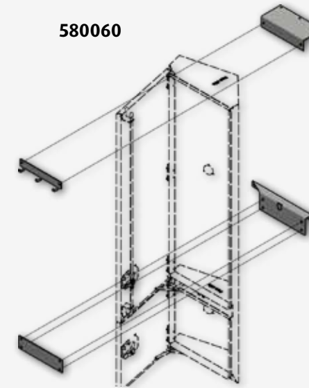
KONSOL Rostfri BevoBox™ höger Scania
