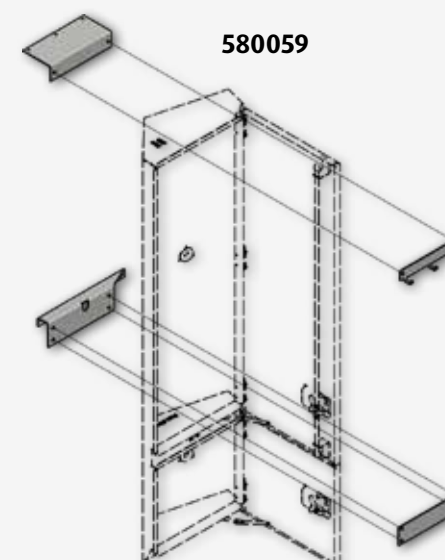
KONSOL Rostfri BevoBox™ vänster Scania
