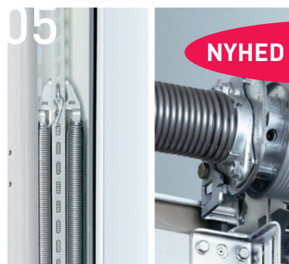
Trækfjederssystem
