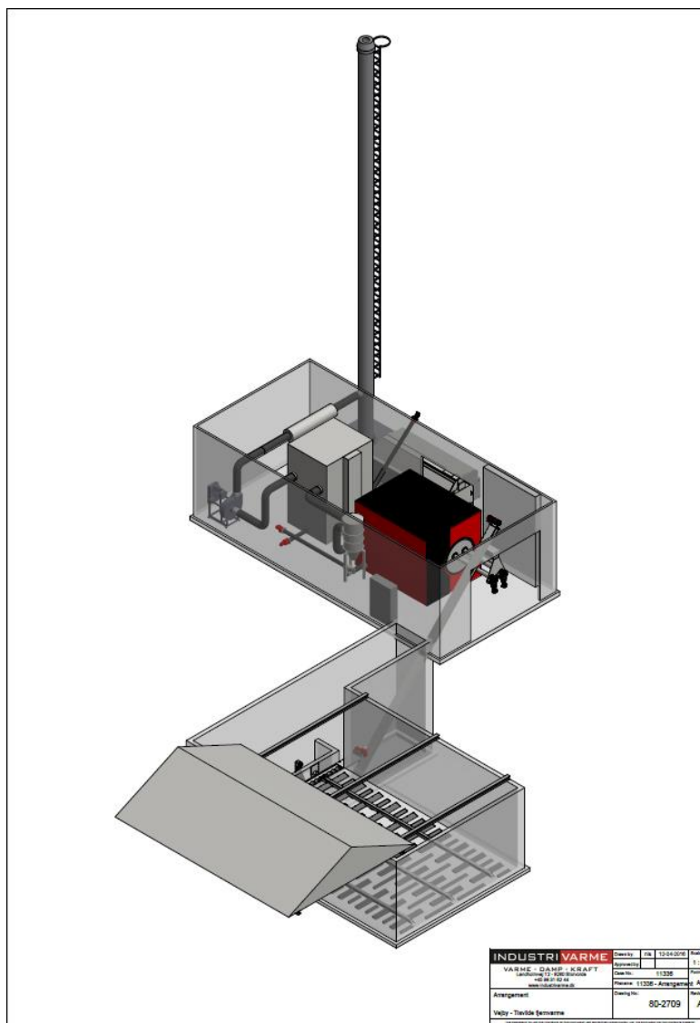
Figur 1: Billedet herover viser INDUSTRIVARMES 3D-tegning af det nye biomasseanlæg.
