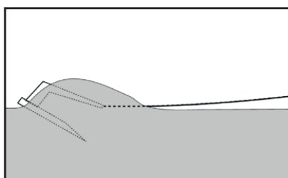
Dregging av anker. Bunnen er for hard for korrekt penetrering
