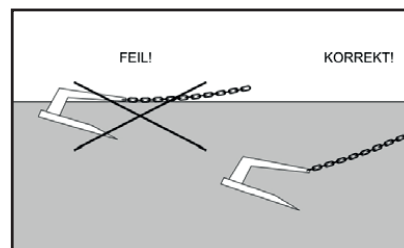
Korrekt penetrering av bunnsediment.
