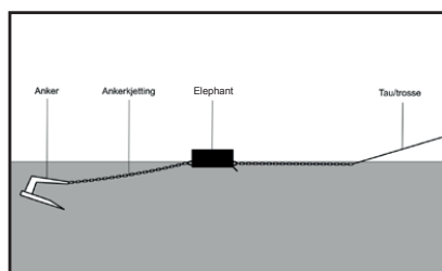
Viser bruk av Elephant foran anker.
