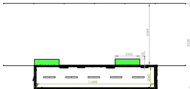
SECTION B-B SCALE 1 : 70
