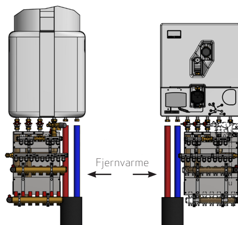
Sammenkobling med systemenheder, hhv. fordelerenhed Compact (tv.) og Slimline (th.).
