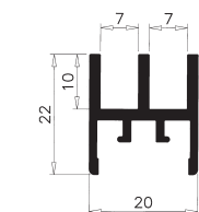
1105-13 Skydedørsprofil. Uafkor- tede længder a 5 m.
