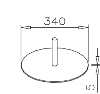
WSF-44 Fodplade med dorn. Ø340mm
