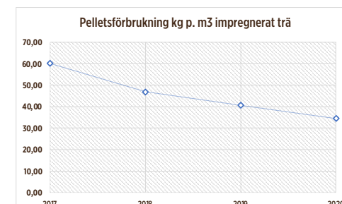
Biogränsle - kWh per m3 impregnerat trä. Nyckeltal inkluderar förbrukning i samtliga processer.
