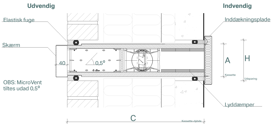
Skærmtype A: MicroVents standardskærm placeres vandret og skjuler diskret ventilationsløsningen.
