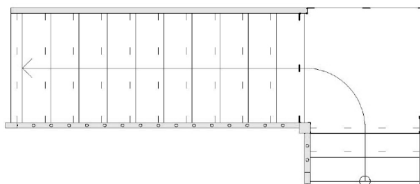
T-13 kvartsvingstrappe med repos
