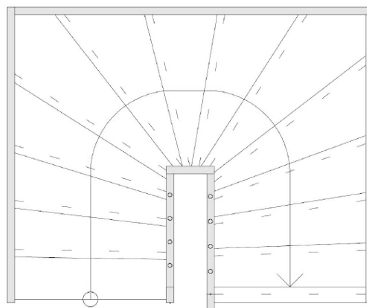
T-15 halvsvingstrappe
