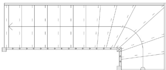
T-12 kvartsvingstrappe
