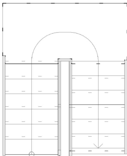
T-14 halvsvingstrappe med repos
