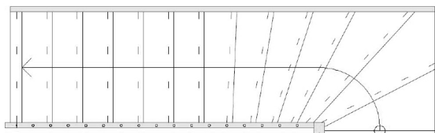
T-11 kvartsvingstrappe
