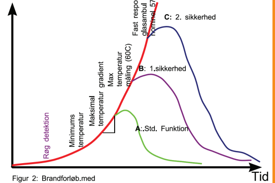
Figur 2: Brandforløb, med A: Standard system aktivering. B: Udløsning uden aktivering af røgmelder C: Uden elektrisk system aktivering
