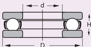
Enkelverkande Yksisuuntaiset Enkeltvirkende
