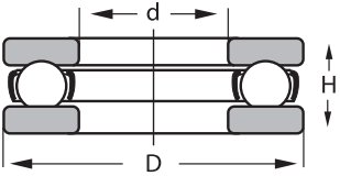
Enkelverkende Yksisuuntaiset Enkeltvirkende
