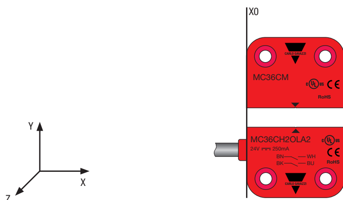
Fig. 2 - Drift og justeringsretning af sensorer
