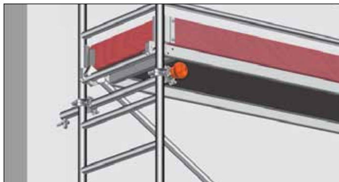
Detalje B
