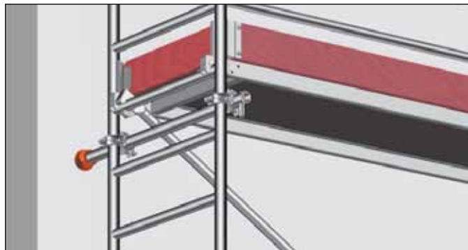
Detalje A
