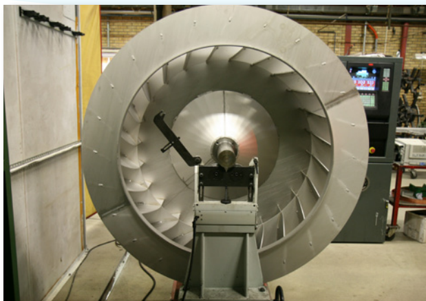
"B hjul" Böjda skovlar med mellanbricka och nav i rostfritt syrafast material.
