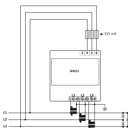
Fig. 10 Trefaset uden neutral (3-ledere)
