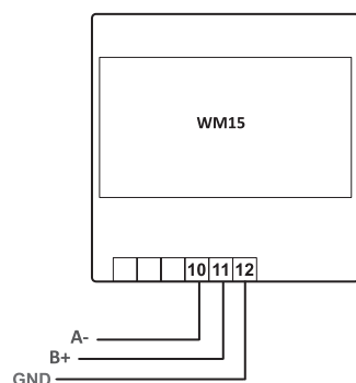
Fig. 14 RS485-port
