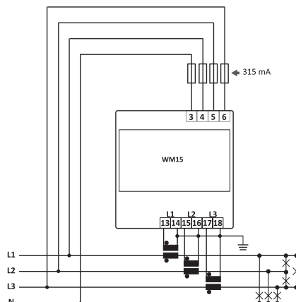
Fig. 11 Trefaset med neutral (4-ledere)
