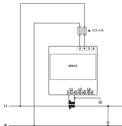
Fig. 9 enkelt-faset (2 ledere)
