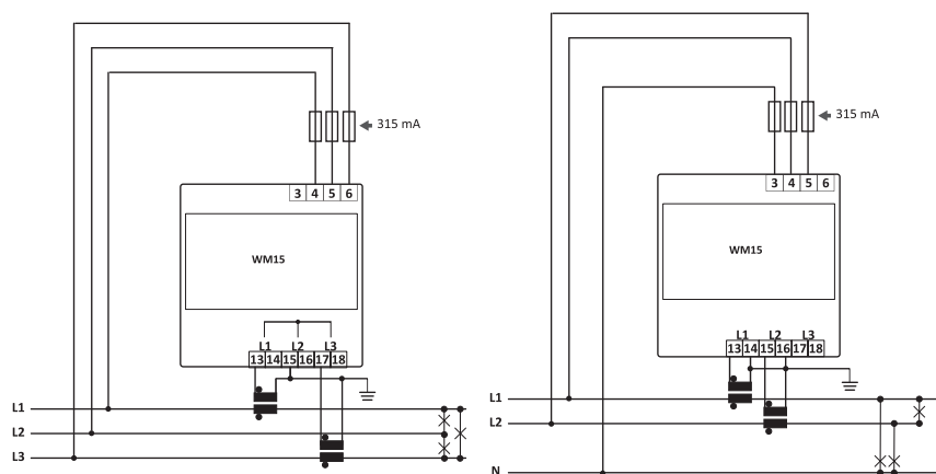
Fig. 7 Trefaset uden neutral (3-le-dere)
