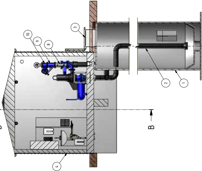
A-A ( 1 : 40 )
