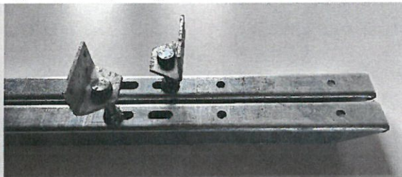
beslag til montering i panelkant kan vendes
