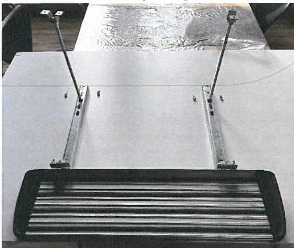
Underside af trin med flytbare gevind
