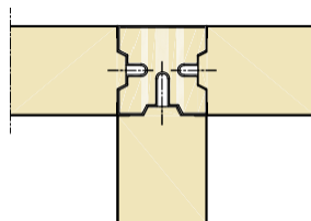
ISO 08 - 10 - 14 - 18 Indvendig væg/Indvendig væg-loft
