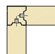
ISO 08 - 10 - 14 - 18 Indvendig væg/Indvendig væg-loft
