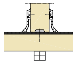
* ISO 06 - 08 - 10 Med gulv+ skillevæg
