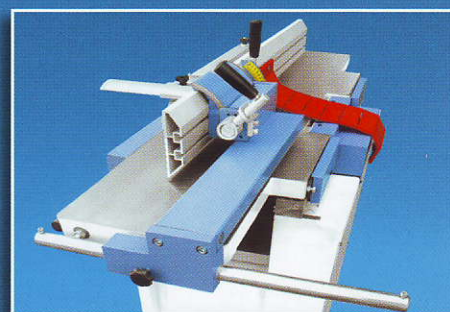
Професионален страничен линеал Profi Seitenabrichtanschlag Professional side fence
