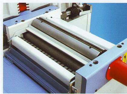
Ножов вал • Messerhobelwelle Cutter block
