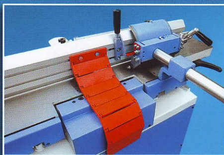
Професионален линеал Profi Abrichtanschlag Professional fence
