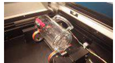
Roterende aggregat For opspænding af krus m.m.
