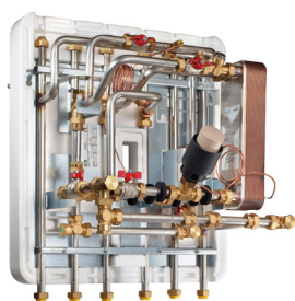
METRO system 2 er en væghængt unit med gennemstrømningsvandvarmer samt direkte fjernvarme til rumvarme. For at overholde DS469 kræves styring af fremløbstemperatur til rumopvarmning på anlægget.
