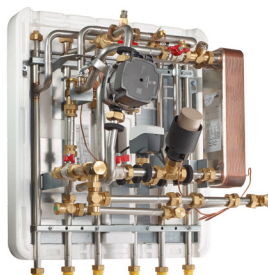
METRO system 4 er en væghængt unit med gennemstrømningsvandvarmer samt direkte fjernvarme med blandesøjfe, trykdifferensregulator og temperaturstyret ventil til rumvarme. Fjernvarmevandet cirkulerer via blandesøjfen, som er integreret i unitten.
