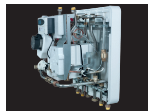
Kabinettet er taget helt af. Nu kan der udføres fuld service.
