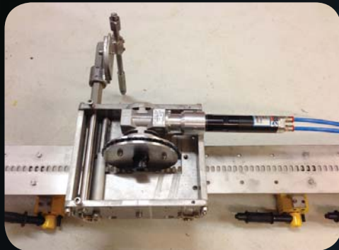
Flexiskinne med skjærevogn. Pneumatisk drift. Festes med magnet, klemmer eller stropper.
