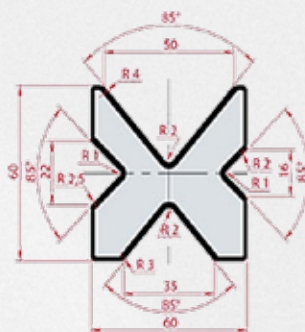
Promecam Underværktøj
