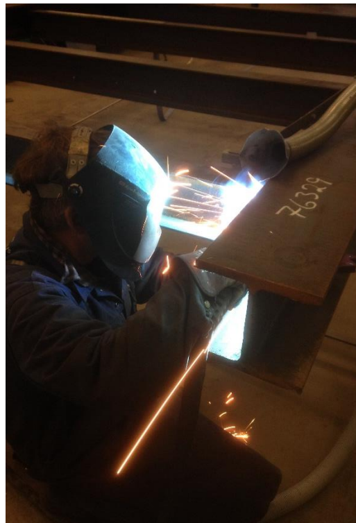
Billede 4: Stålkonstruktioner fremstilles af vores smede som udfører certifikatsvejsning efter EN1090.
