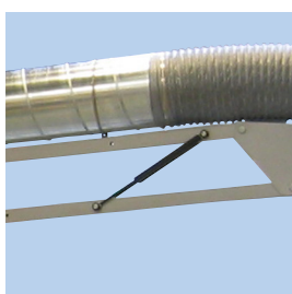
Gasfjeder Arm afbalanceret med gasdæmpere.
