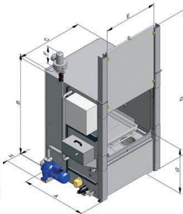
Typ P: Tvättmaskin med pneumatisk lucka
