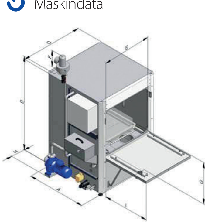
Typ F: Tvättmaskin med fälllucka
