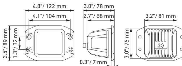
LED Cube 3,2" (til indbygning)
