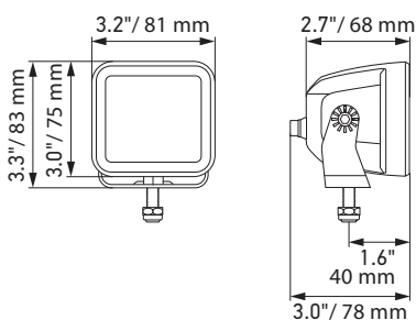
LED Cube 3,2" (til påbygning)
