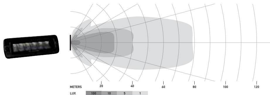
LED Mini Lightbar 6,2", indbygning, bred lysfordeling
