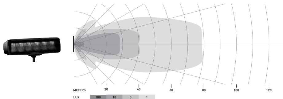
Black Magic Mini Lightbar 6,2", bred lysfordeling
