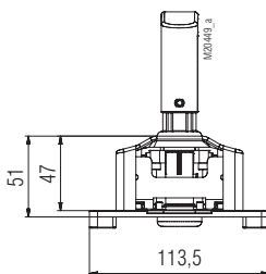
Linke Seitenansicht
