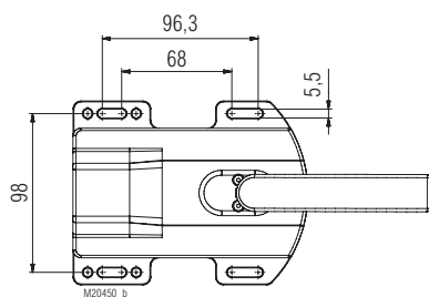
Draufsicht
