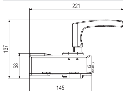
Vorderansicht
