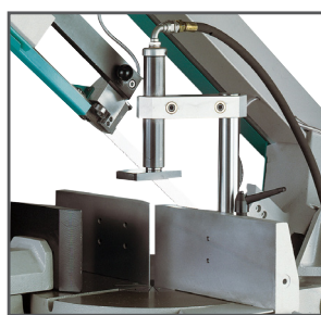
Hydraulisk vertikal skruestik
