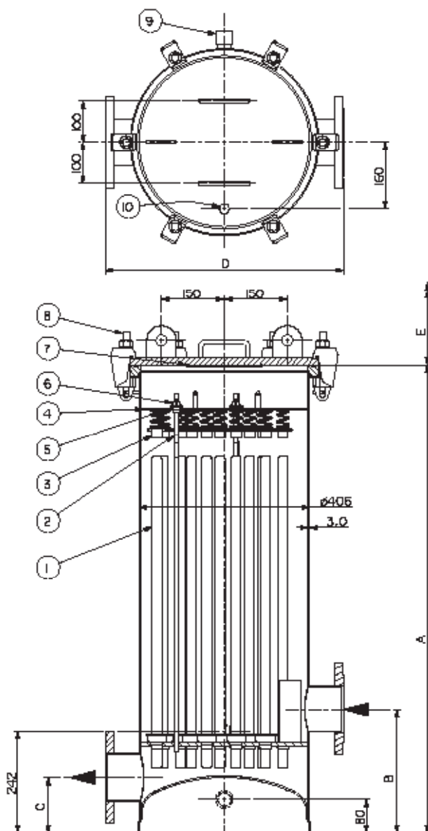
Generell ritning av 6122 serien. Om teknisk ritning av specifikt filter önskas: Kontakta er leverantör.
