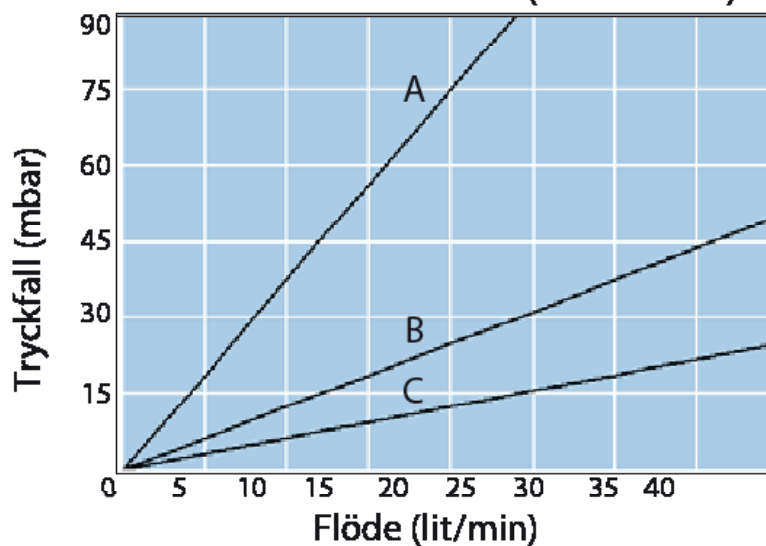
Flödeskurva för vatten (10" element)
