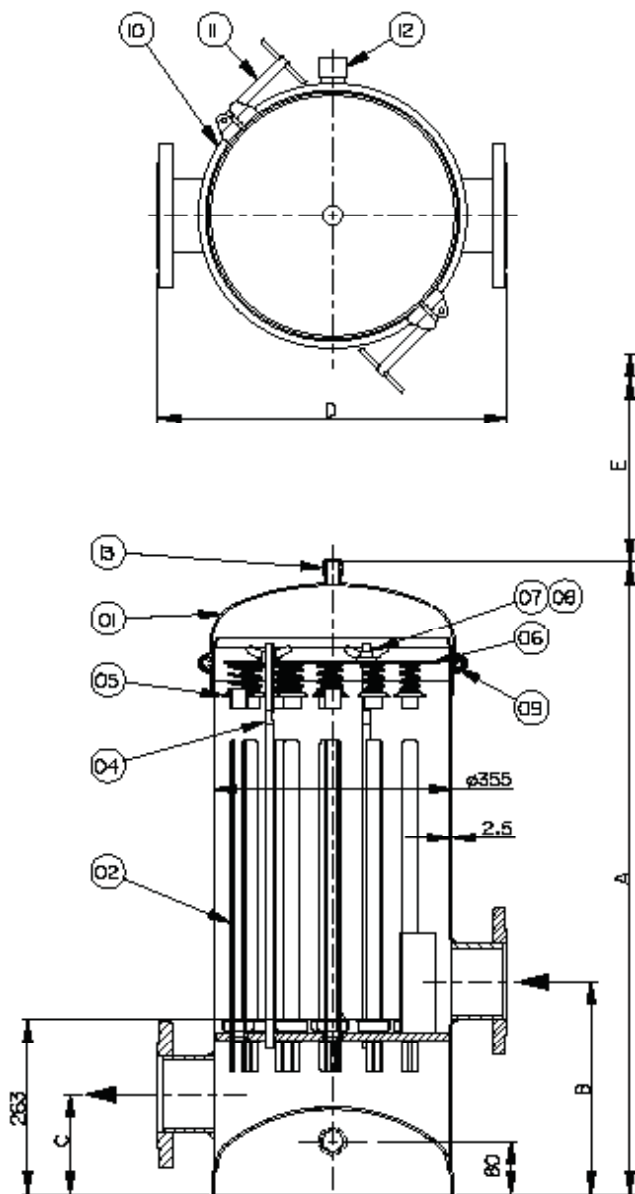
Generell ritning av 6118 serien. Om teknisk ritning av specifikt filter önskas: Kontakta er leverantör.
