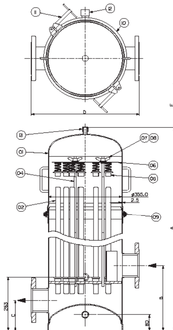
Generell ritning av 6315 serien. Om teknisk ritning av specifikt filter önskas: Kontakta er leverantör.
