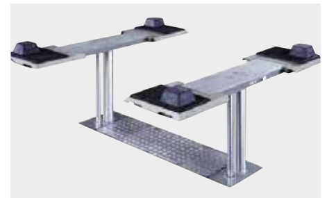
2-stemplet undergulv løfter
