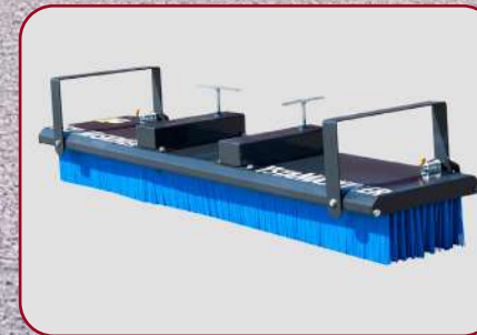
Sopborste YB-245 med gaffelfäste och uppfällbara stödben
