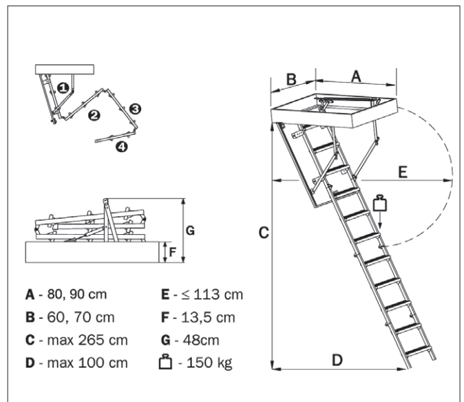
Varmeisoleret loftlem af "sandwich-typen" med en tykkelse på 46 eller 86 mm. Isoleret med polystyren, dobbeltsidet, beklædt på begge sider med hvid HDF-plade og med tætningsliste.
