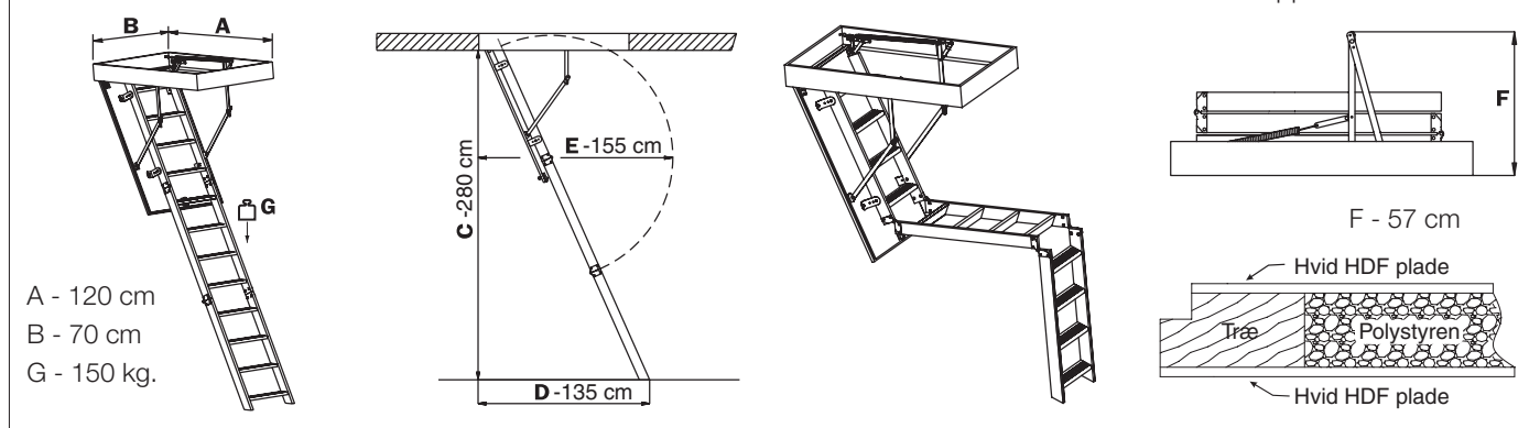
Sandwich lofttrappekonstruktion
