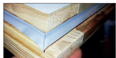
Sandwich lofttrappekonstruktion
