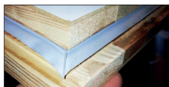
Varmeisoleret loftlem af "sandwich-typen" med en tykkelse på 46 eller 86 mm. Isoleret med polystyren, dobbeltsidet, beklædt på begge sider med hvid HDF-plade og med tætningsliste.
